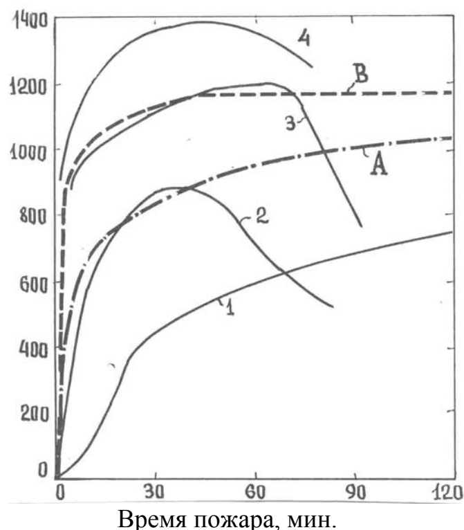
Рис. 1.2 Характерные температурные режимы пожаров на объектах различного назначения
